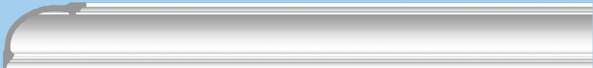
DWL 1003A DWL 1012A /B: 18 /H: 15 /L:225 /Kg: 9,8 /Stück: 89,10 € /Meter: 39,60 € Netto Anschluss: DWL 1003
