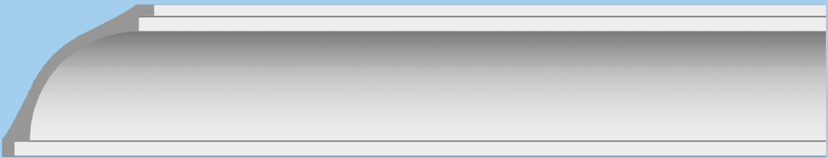
DWL 3016D /B: 18 /H: 18 /L: 225 /Kg: 9,8 / Stück: 97,20 € Meter: 43,20 € Netto
