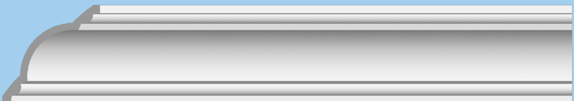
DWL 3014H /B: 18 /H: 18 /L: 225 /Kg: 9,20 /Stück: 97,20 € /Meter: 43,20 € Netto
