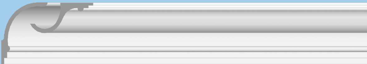
I 001AB /B: 30 /H: 20 /L:225 /Kg: 19,1 /Stück: 173,34 € /Meter: 77,04 € Netto
