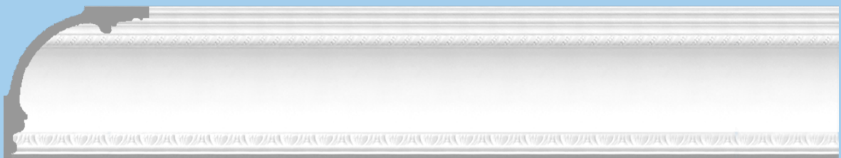
DWL 1008A /B: 22,5 /H: 20,5/L: 123 /Kg: 7,1 /Stück: 63,47 € / Meter: 51,60 € Netto Anschluss: DWL1008
