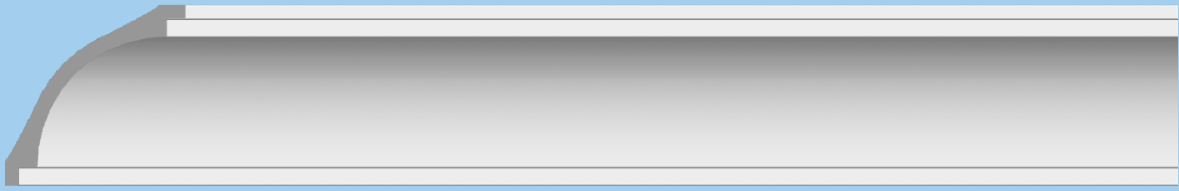
DWL 3016C /B: 15 /H: 15 /L: 225 /Kg: 7,6 / Stück: 81,00 € Meter: 36,00 € Netto
